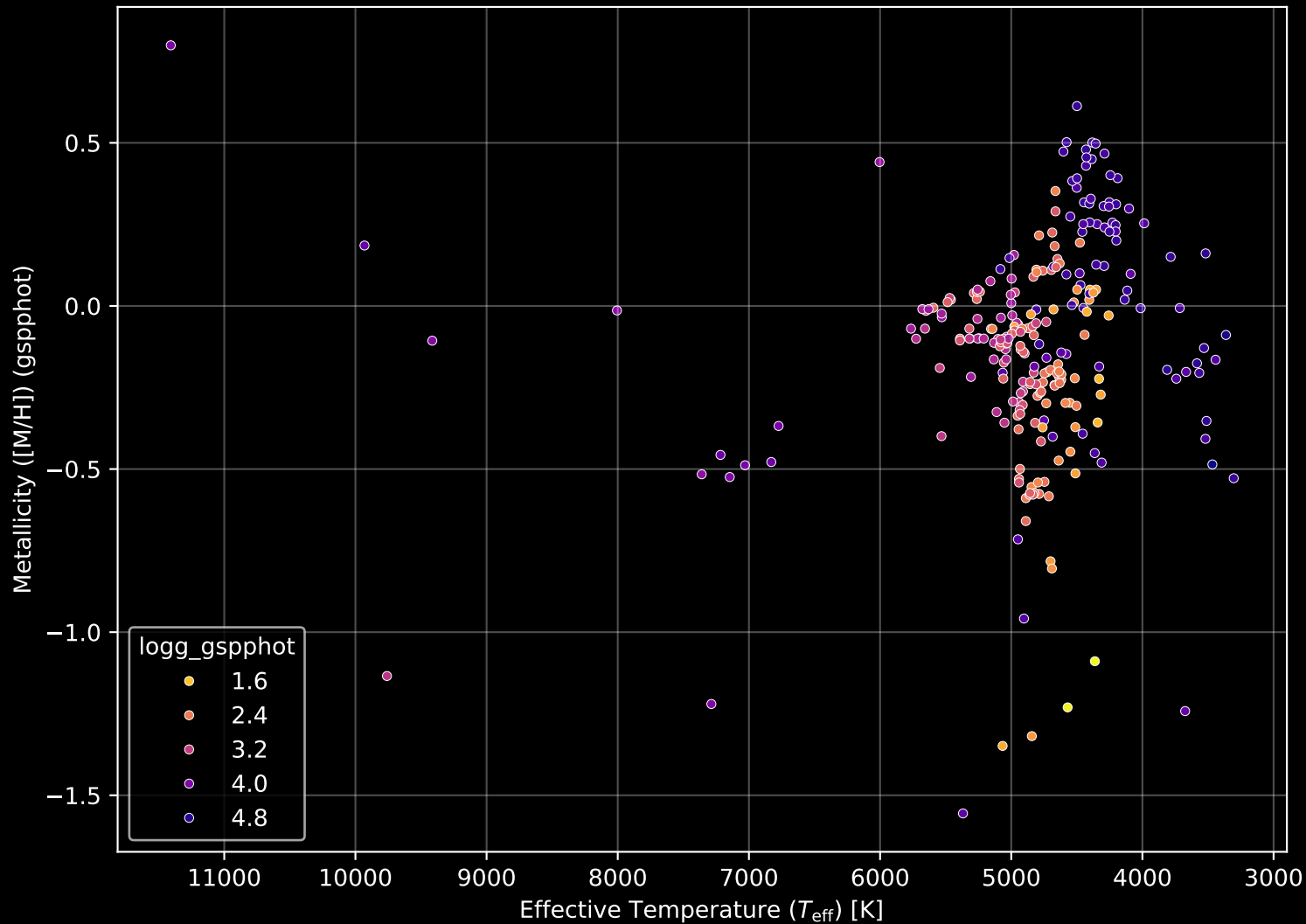
APOGEE DR17 Field: [139+27_btx] Stellar Population Parameters (n= 259)
